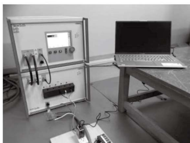
雷サージ耐性評価試験
