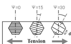
ii) 引張応力が作用している状態 \Psi が大きい結晶 d が大きい
