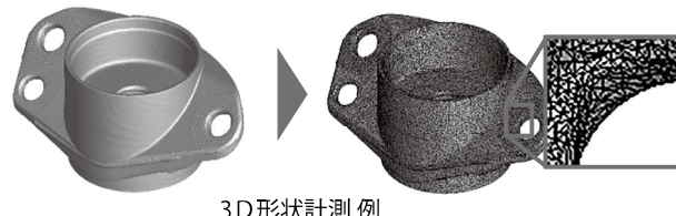
3D 形状計測 例
