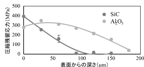
図3 深さ方向に対する応力分布
