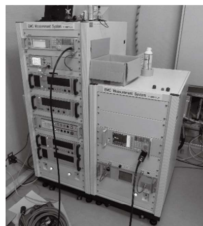
ラージループ測定
