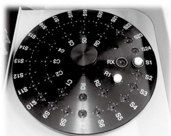
図. サンプルチェンジャ (最大24試料)
