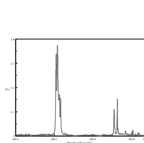
図1 赤外吸収スペクトル
