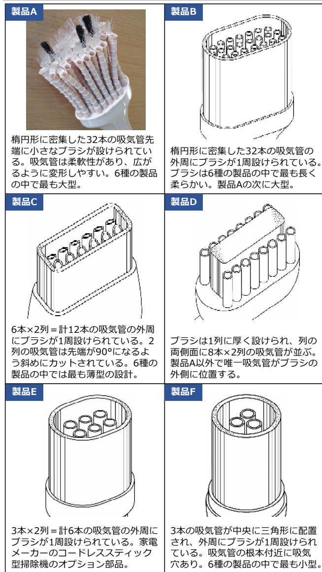
図3 類似製品の設計面の特徴
