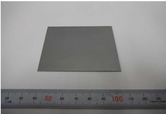
金属の中性塩水噴霧サイクル試験前
