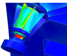
フレームの補強効果確認
