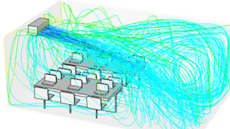
居室内における空調効果確認
